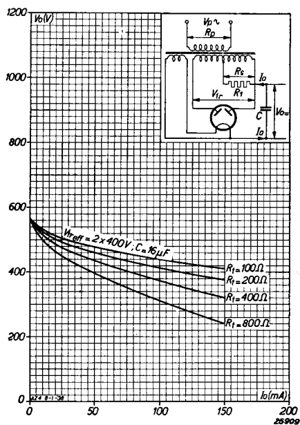
Belastingkromme van de AZ 4 bij een secundaire spanning van den voedingstransformator van 2 \times 400 V en verschillende inwendige weerstanden R_{tot} = R_1 + R_s + u^2 R_p .
