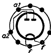
Sockelschaltchema
