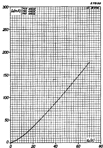
Abb. 3 Anodenstrom pro Anode als Funktion der angelegten Gleichspannung.
