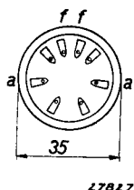
Abb. 2 Elektrodenanordnung und Sockelanschlüsse.
