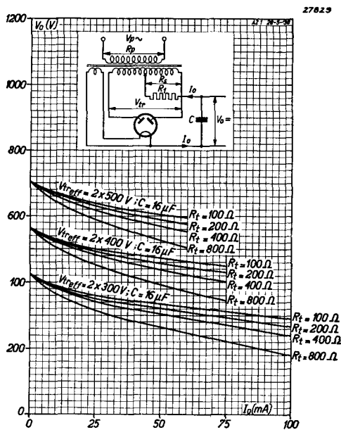
Abb. 4 Belastungskurven bei verschiedenen Transformatorleerlaufspannungen und Innenwiderständen des Transformators ( R_t = R_s + u^2 R_p + R_l ).
