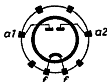
Sockelschaltschema
