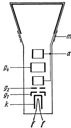
Aufbauschema der Röhre
