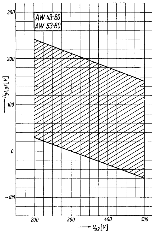
Dg. 121. Zaostřovací napětí U_{g3,g5} v závislosti na napětí stínicí mřížky U_{g2} pro optimální zaostření uprostřed stínítka. Katodový proud I = 100 \mu\text{A} a napětí hlavní anody U_{a,g4} = 15 \text{ kV} .
