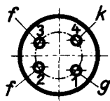
Sockelansicht von unten Bottom view of base Culot vu du bas Casquillo visto desde abajo
