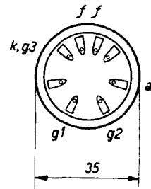
Sockelanschlüsse und Elektroden- anordnung.
