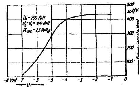
Konversionssteilheit für eine Oszillatorspannung von 2,5 \text{ V eff} in Abhängigkeit von der Spannung U_{g1}
