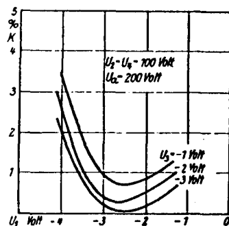
Klirrfaktor für Wechselspannung U_{g1} = 0,5 \text{ V eff} (Außenwiderstand: 5 \text{ k}\Omega )
