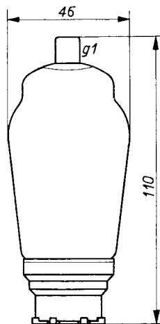
Abb. 4 Abmessungen der Röhre AH 1.
