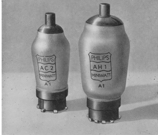
Abb. 2 Die Miskombination einer Regelhexode AH1 als Modulatorröhre mit einer Triode AC2 als Oszillatorröhre.
