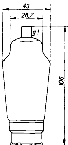
Abb. 4 Abmessungen der Röhre AF 7.
