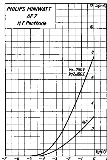
Abb. 2 Anodenstrom und Schirmgitterstrom als Funktion der Steuergitterspannung
