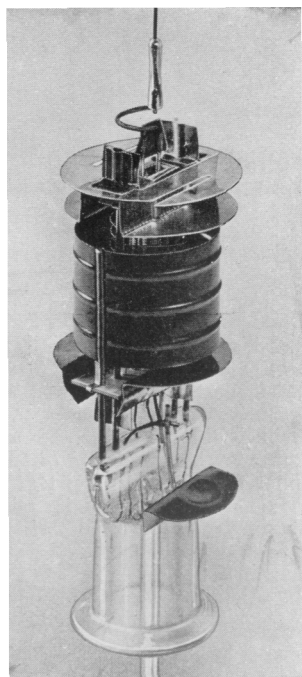
Abb. 1 Innenaufbau der Röhren AF 3 und AF 7.
