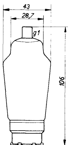
Abb. 1 Abmessungen der Röhre AF 3.
