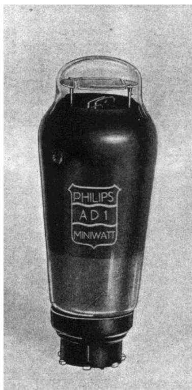
La nouvelle triode de sortie de la série 4 volts à courant alternatif AD1.
