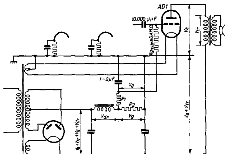
Montage d'une résistance ( R_f ) en série avec la self de filtrage de l'alimentation plaque pour obtenir une polarisation semi-automatique du tube de sortie à chauffage direct. Pour la signification des indices, voir la figure 7. La tension continue aux bornes du premier condensateur de filtre devra être égale à V_g + V_{dr} + V_g + V_{dr} . La polarisation négative du tube de sortie ne se retrouve pas, dans ce cas, entre cathodes et filaments des tubes à chauffage indirect du poste.
