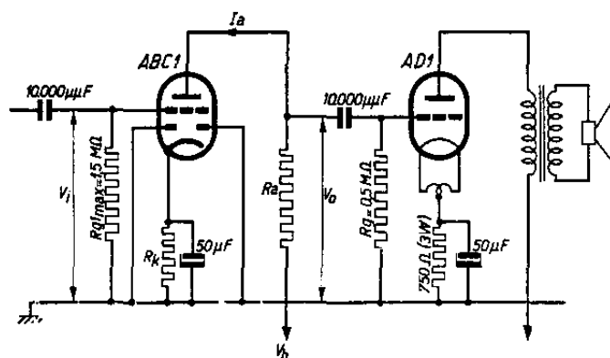
Montage du tube ABC 1 (ou AC 2) comme tube préamplificateur devant la triode de sortie AD 1 utilisée comme amplifiatrice de sortie en classe A. Fig. 11
