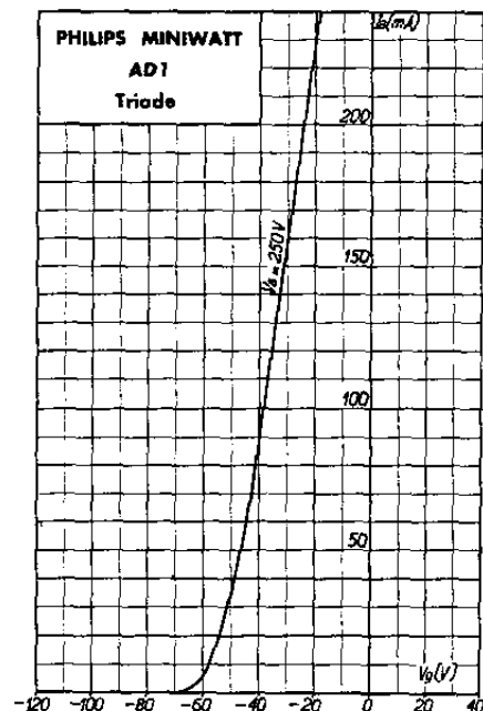
Courant d'anode en fonction de la tension négative de la grille pour V_a \approx 250 volts.
