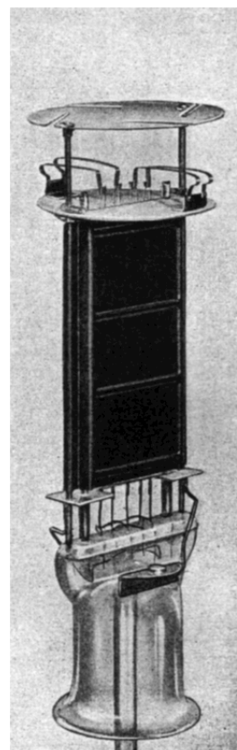
Construction intérieure de la triode de sortie AD 1.
