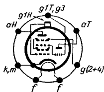
Sockelschaltschema
