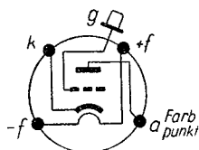
Schaltschema
