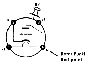
Sockelschaltbild Base connection
