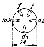
Abb. 3 Elektrodenanschlüsse am Sockel der Röhre AB 2.
