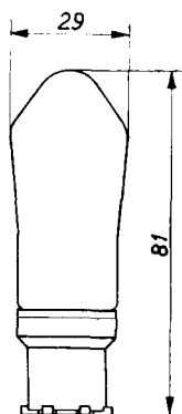
Abb. 4 Abmessungen der Röhre AB 2.
