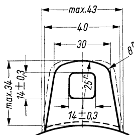
Einzelheit „C“
