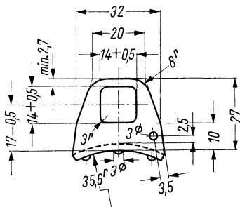
Einzelheit „C“
