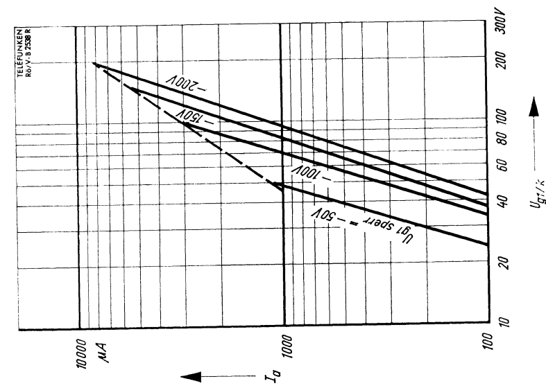
Gittersteuerung · Grid control I_a = f(U_{g1/k}) Diagramm 2
