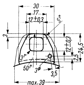
Einzelheit „C“
