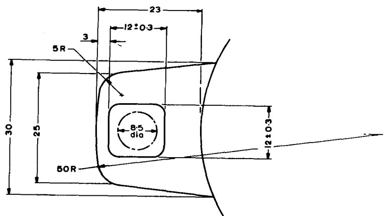
Mounting lug
