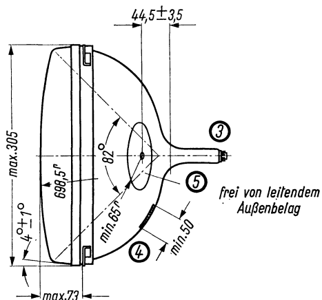
Schnitt A-B
