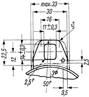
Einzelheit „C“
