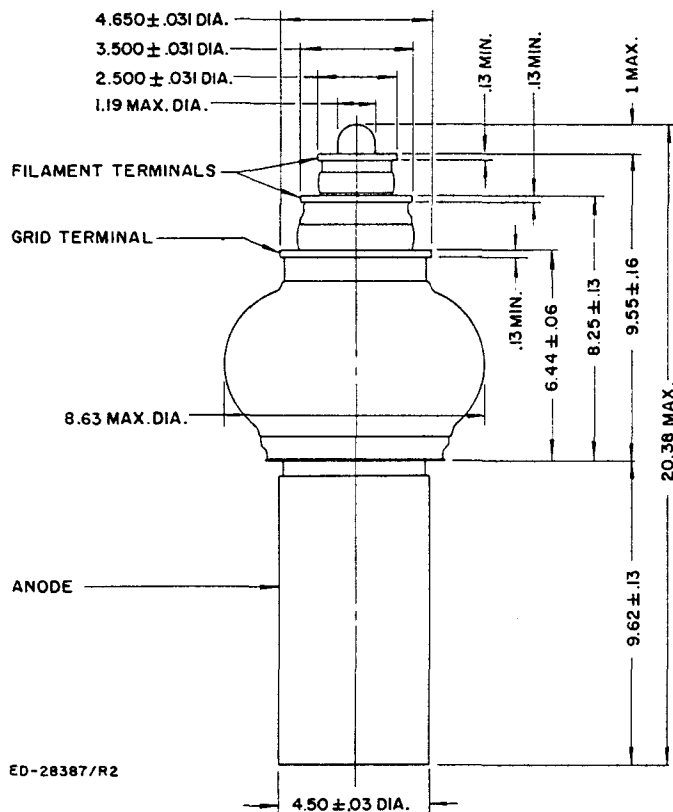
DIMENSIONS — ML-8038
