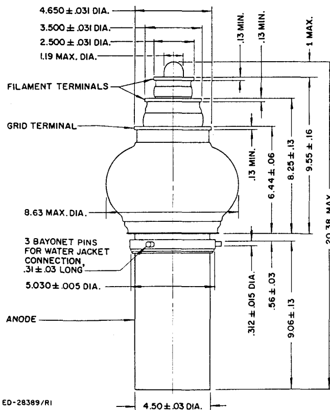
DIMENSIONS — ML-8041
