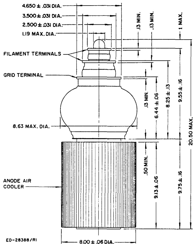
DIMENSIONS — ML-8038
