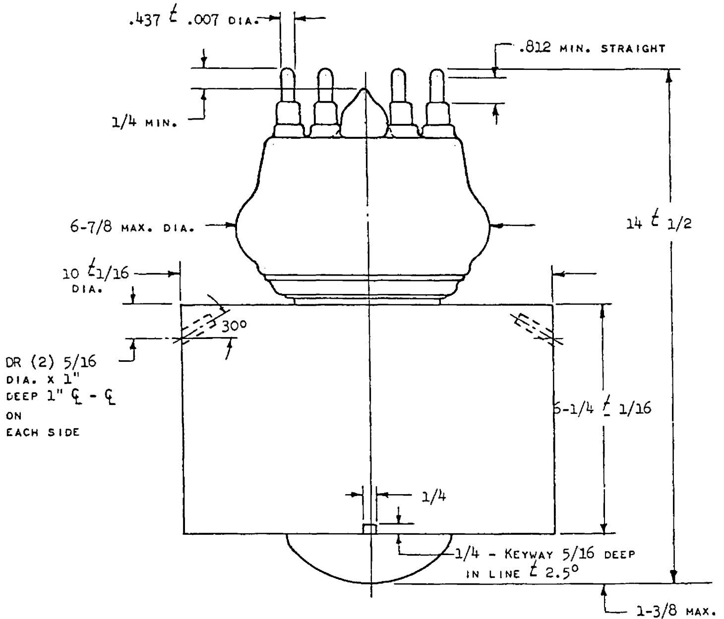
F-7328 POWER TRIODE
