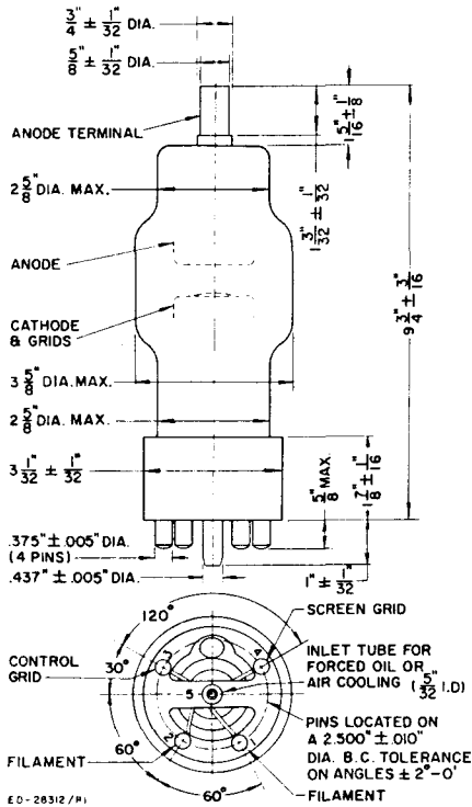
DIMENSIONS — ML-7248
