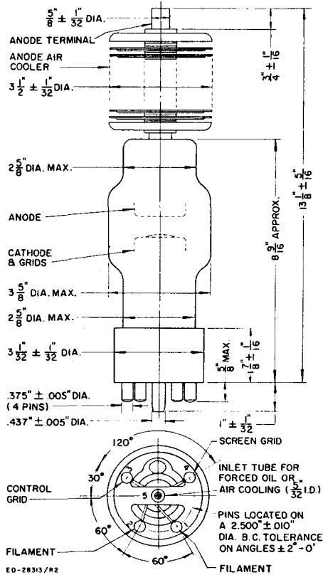
DIMENSIONS — ML-7249
