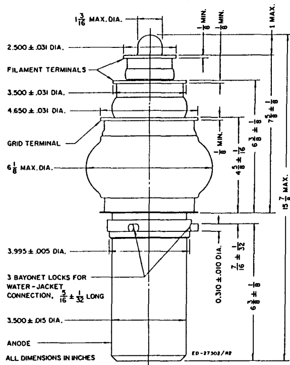
DIMENSIONS — ML-7124
