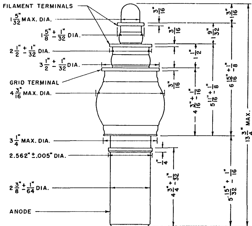
DIMENSIONS — ML-7120
