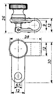
Heizer connector Connecteur de filament Heizfadenklemme 40634
