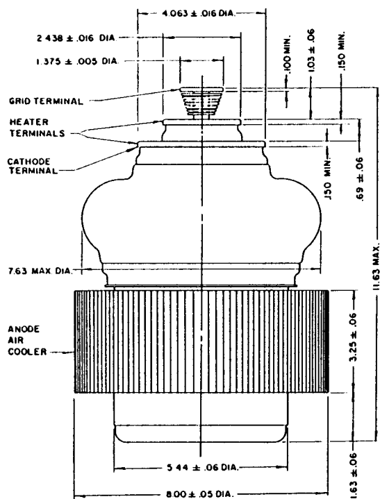
DIMENSIONS — ML-7715
