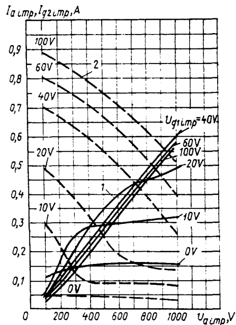
Усредненные импульсные характеристики: 1 — анодные; 2 — сеточно-анодные (по сетке второй) U_h = 6.3 V, U_{g2} = 300 V, \tau = 2 \mu s, f = 100 Hz Averaged pulse characteristics: 1 — anode; 2 — grid-anode (for grid 2) U_h = 6.3 V, U_{g2} = 300 V, \tau = 2 \mu s, f = 100 Hz
