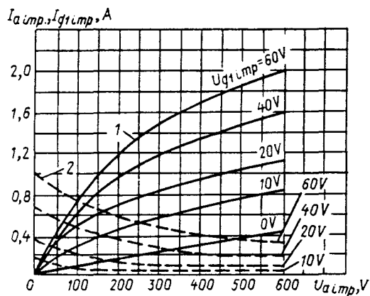
Усредненные импульсные характеристики: 1 — анодные; 2 — сеточно-анодные (по сетке второй) U_h = 6.3 V, U_{g2} = 300 V, \tau = 2 \mu s, f = 100 Hz Averaged pulse characteristics: 1 — anode; 2 — grid-anode (for grid 2) U_h = 6.3 V, U_{g2} = 300 V, \tau = 2 \mu s, f = 100 Hz
