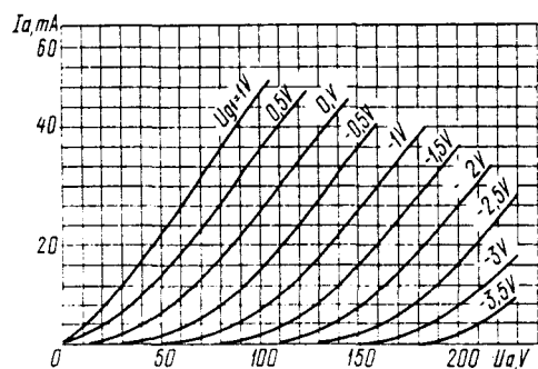
Усредненные характеристики (триодное включение)
