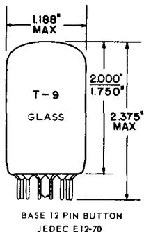
OUTLINE JEDEC 9-58
