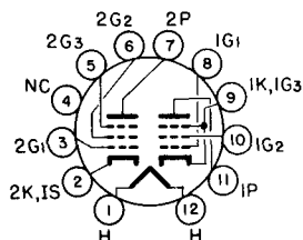
BASING DIAGRAM JEDEC 12EZ
