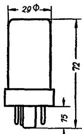
Kolbenabmessungen
