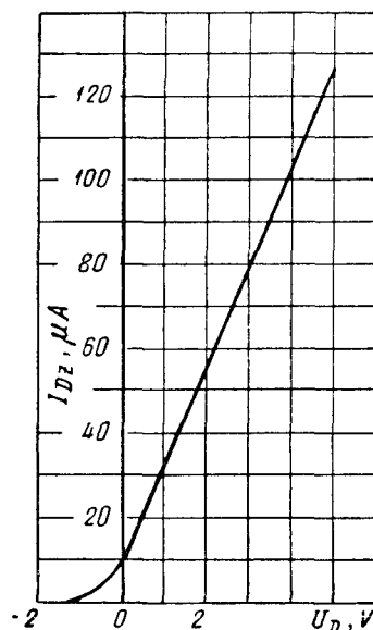
I_{DZ} = f(U_D) (для одного диода) (for one diode) U_h = 6,3 V R_a = 40 k \Omega
