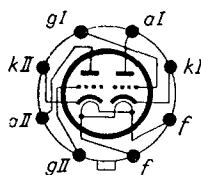
Sockelschaltschema
