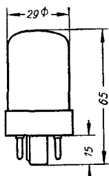
Kolbenabmessungen
