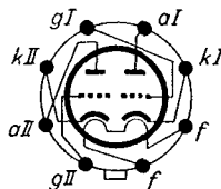
Sockelschalt-schema
