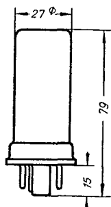
Kolbenabmessungen
