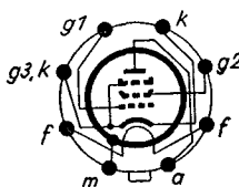
Sockelschaltsschema
