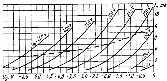
I_a = f(U_g)
