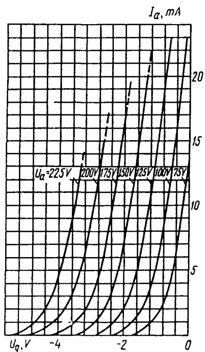
Усредненные анодно-сеточные характеристики U_h = 6,3 \text{ V}
