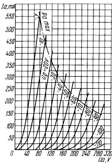
Усредненные анодные характеристики (при работе с одним катодом): U_i = 6,3 \text{ В} ; — — — наибольшая допустимая мощность, рассеиваемая анодом ( P_{a \text{ max}} ) Averaged Anode Characteristic Curves (single-cathode operation): U_i = 6.3 \text{ V} ; — — — P_{a \text{ max}}
