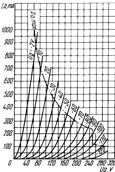
Усредненные анодные характеристики: U_i = 12,6 \text{ В} ; — — — наибольшая допустимая мощность, рассеиваемая анодом ( P_{a \text{ max}} ) Averaged Anode Characteristic Curves: U_i = 12.6 \text{ V} ; — — — P_{a \text{ max}}
