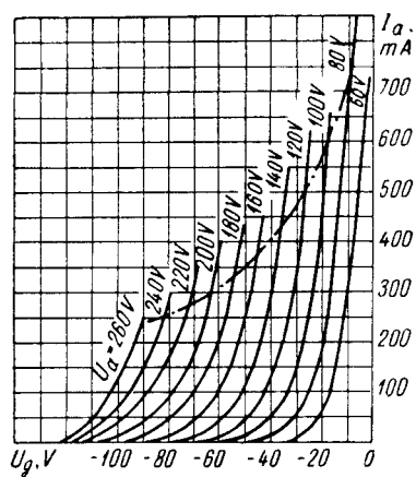
I_a = f(U_g) — · — · — P_{a \max} U_h = 12,6 \text{ V}
