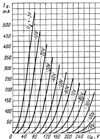
I_a = f(U_a) (при работе с одним катодом) (when using one cathode) — · — · — P_{a \max} U_h = 6,3 \text{ V}
