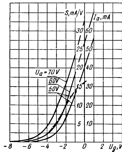
I_a, S = f(U_g) \text{—} I_a U_h = 6,3 \text{ V} \text{---} S
