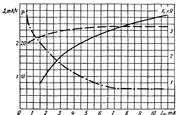
S, \mu, R_i = f(I_a) (каждого триода) (for each triode) — S U_h = 6,3 \text{ V} - - - \mu U_a = 250 \text{ V} - · - · - R_i
