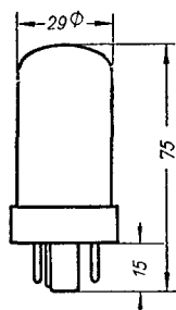
Kolbenabmessungen
