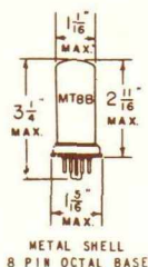
6N7
