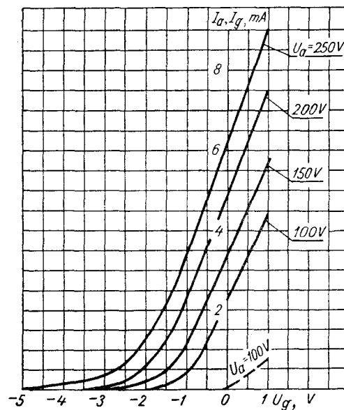
I_a, I_{gT} = f(U_{gT}) (каждого триода) (for each triode) — I_a U_h = 6,3 \text{ V} - - I_{gT}
