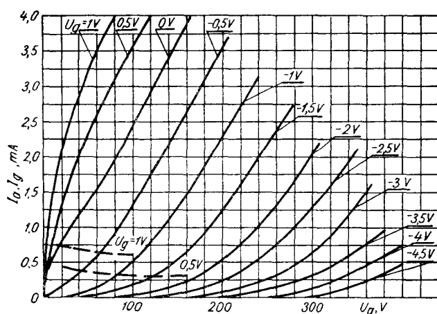
I_a, I_{gT} = f(U_a) (каждого триода) (for each triode) — I_a U_h = 6,3 \text{ V} - - I_{gT}
