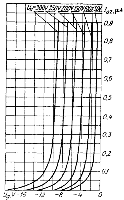
I_{a2} = f(U_{gT}) (каждого триода) (for each triode) U_h = 6,3 \text{ V}
