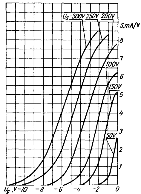
S = f(U_{gT}) (каждого триода) (for each triode) U_h = 6,3 \text{ V}
