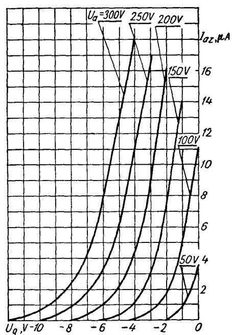
I_{az} = f(U_{gT}) (каждого триода) (for each triode) U_h = 6,3 \text{ V}
