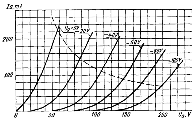
I_a = f(U_a) (каждого триода) (for each triode) — — — P_{a \max} U_h = 6,3 \text{ V}
